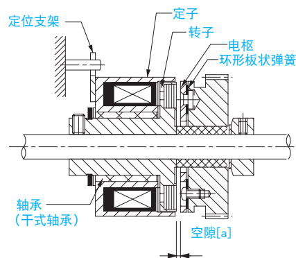
轴承安装型（干式轴承）构造
