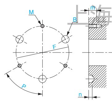
电枢 3 型安装尺寸
