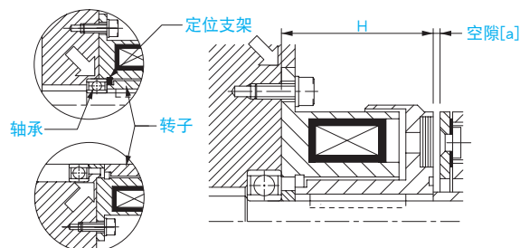
定子・转子的安装（法兰安装型）
