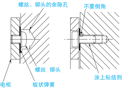
电枢 3 型安装的图
