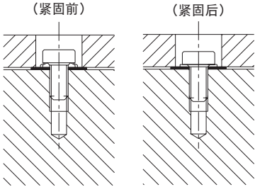
弹簧垫的使用方法
