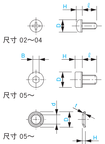
电枢 3 型安装部件
