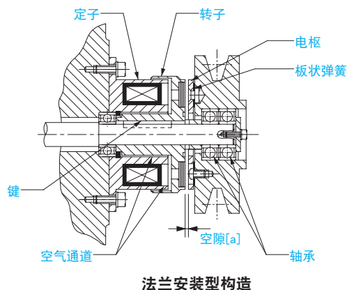
法兰安装型构造
