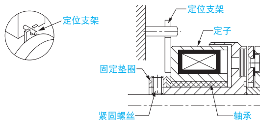
定子・转子的安装（轴承安装型）
